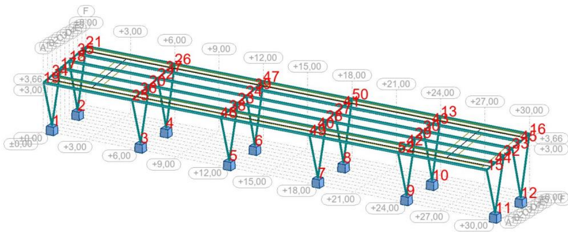
Slika 26. Prikaz čvorova konstrukcije [3]
