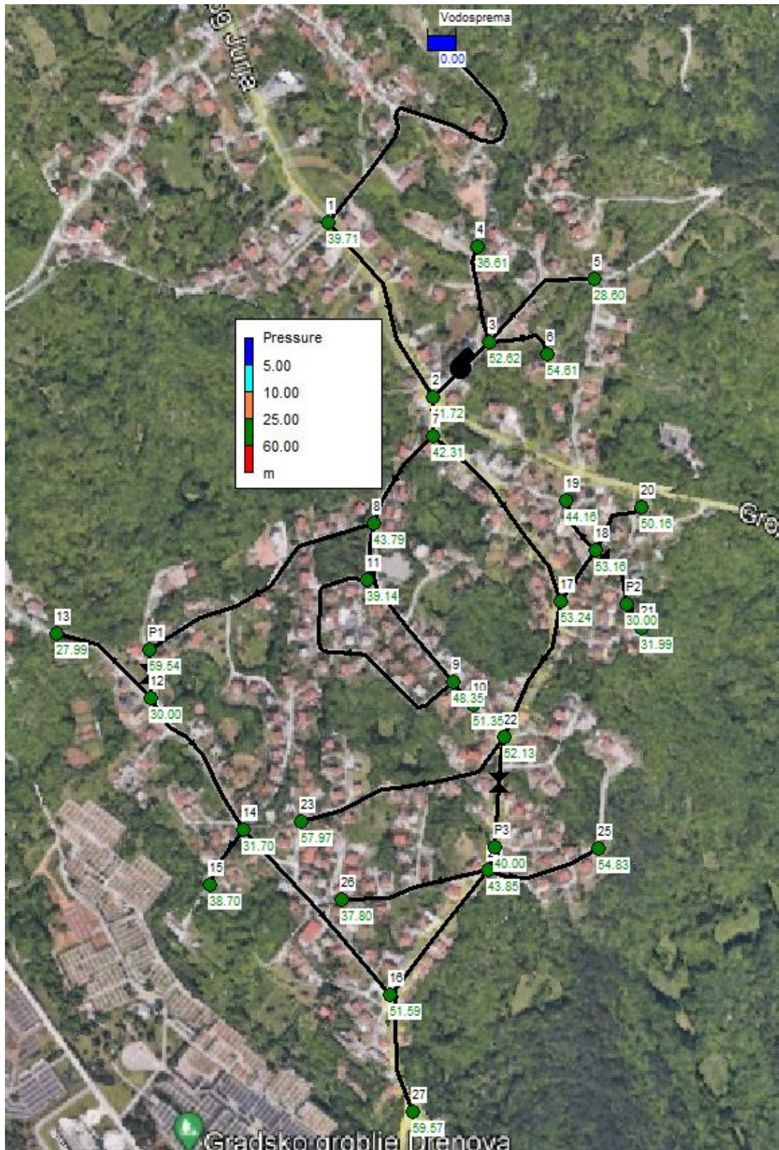
Slika 19: Mreža bez požarnog zahtjeva s redukcijskim ventilima i crpkom
