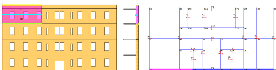
Slika 108. Geometrija pretpostavljenog bloka mehanizma otkazivanja tipa F primjer 10 (lijevo), prikaz položaja zgloba (u sredini), položaj zida u konstrukciji (desno)
