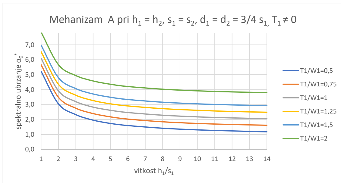
Slika 42. Spektralno ubrzanje za mehanizam otkazivanja A - slučaj 4
