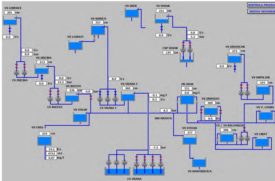
Slika 2.11. Shematski prikaz današnjeg vodoopskrbnog sustava otoka Cres i Lošinja (Institut IGH, 2016,)
