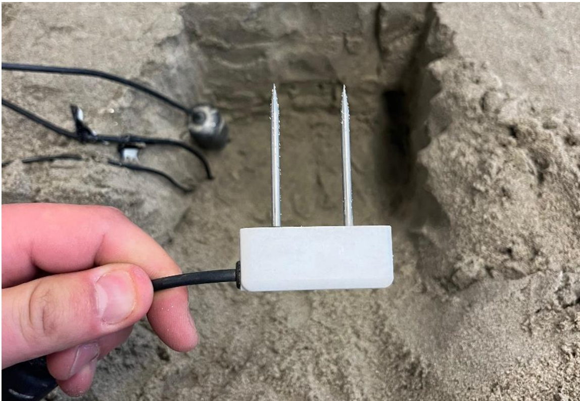
Slika 12: Senzor Teros 10
