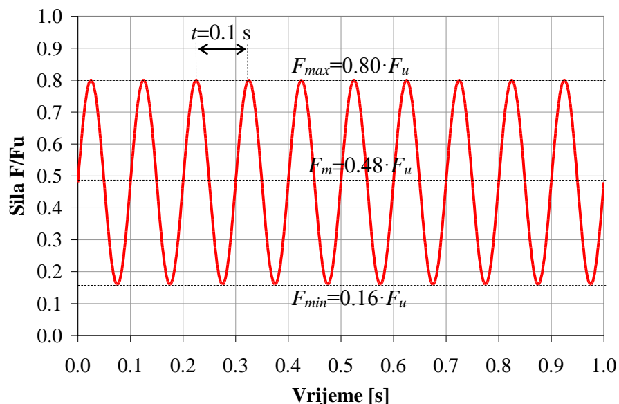
Slika 3.16 Cikličko ispitivanje greda na savijanje u tri točke do sloma pod kontrolom sila
