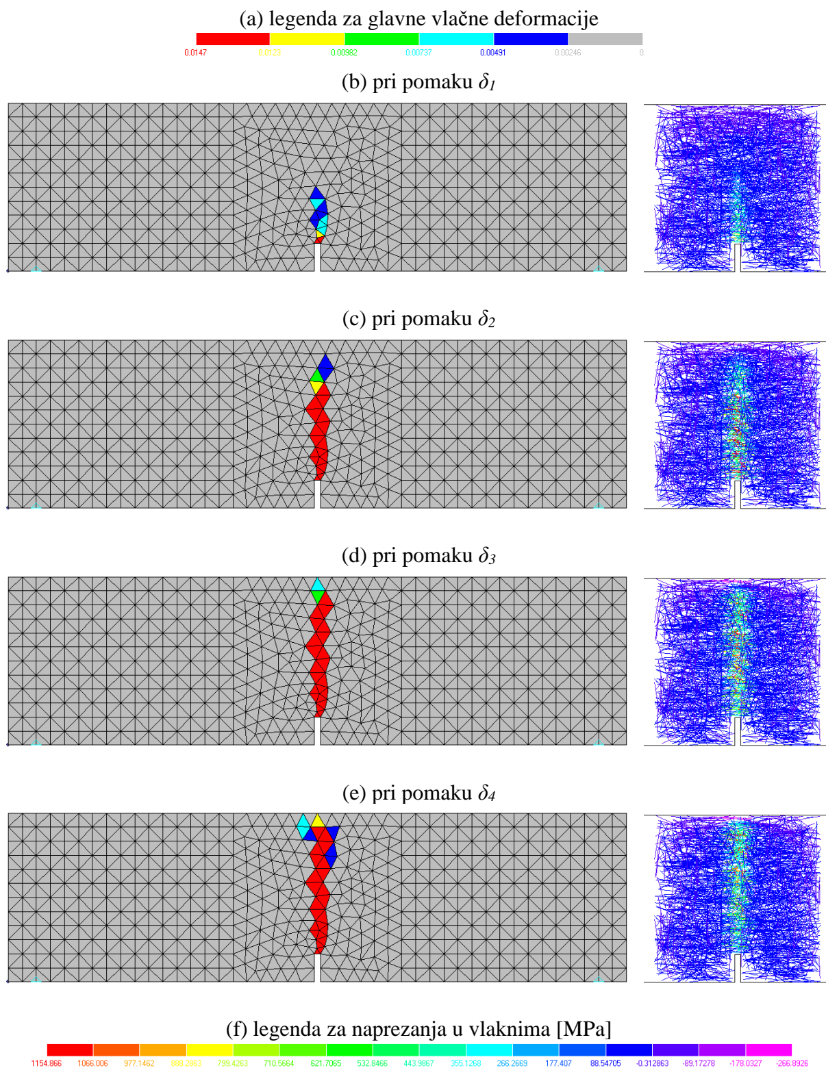
Slika 5.32 Prikaz pukotina (lokalizacija glavne vlačne deformacije) i naprezanja u vlaknima za model M1_05_
