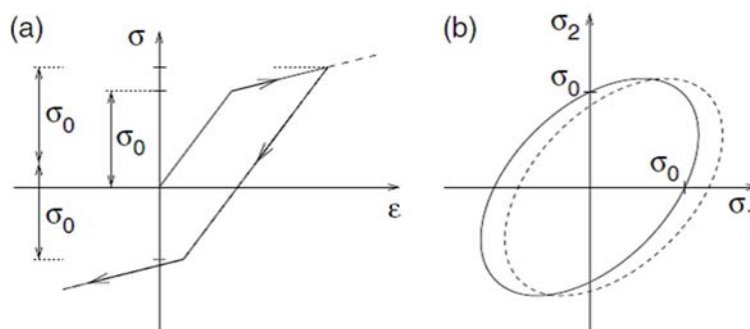
Slika 2.19 Kinematički model očvršćivanja: a) Dijagram naprezanja i deformacije za jednoosno ispitivanje, b) Razvoj plohe popuštanja [54]
