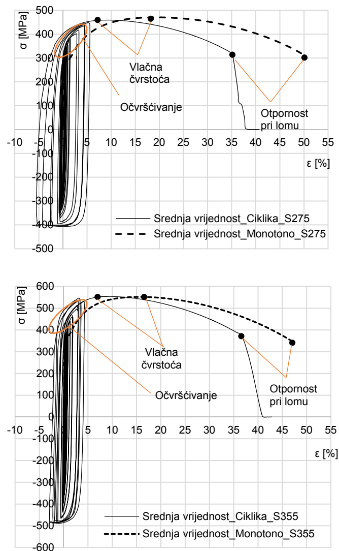
Slika 2.16 Usporedba monotonihih krivulja naprezanja-deformacije i histreznih krivulja za čelike S275 i S355 [38]
