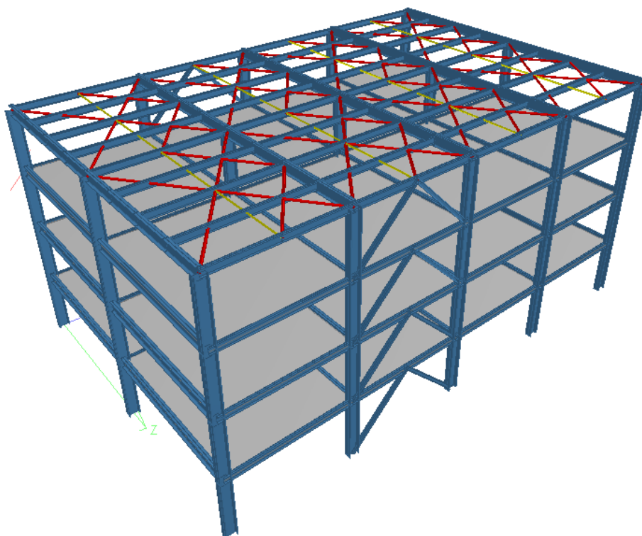
Slika A.1 3D vizualizacija konstrukcije
