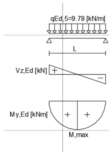
Slika 15: Dijagrami M i V za najveću pozitivnu kombinaciju podrožnice, GSN
