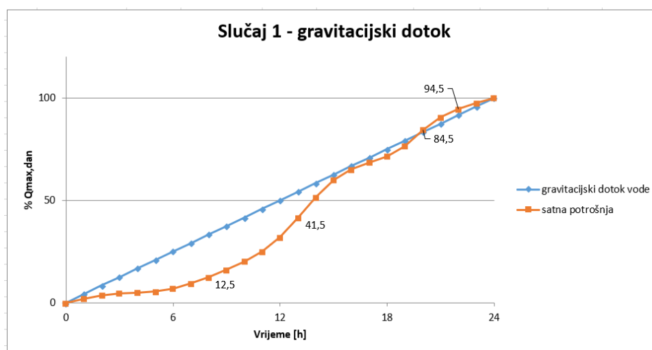
Slika 27. Grafoanalitičko rješenje gravitacijskog dotoka vode u vodospremu
