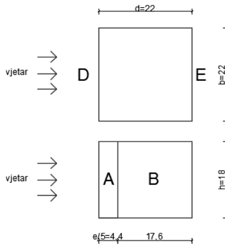
Slika 6: Tlocrt i bočni pogled zgrade s prikazanim vjetrovnim zonama
