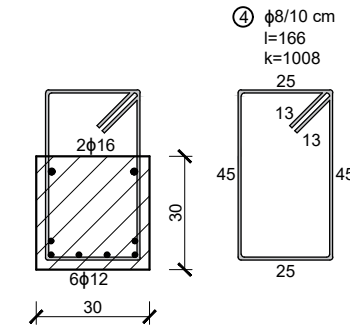
Presjek C-C, M 1:20
