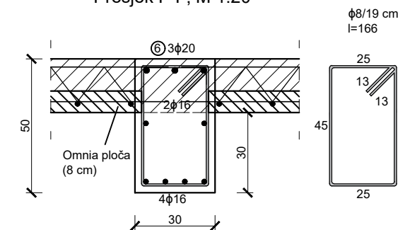
Presjek F-F, M 1:20
