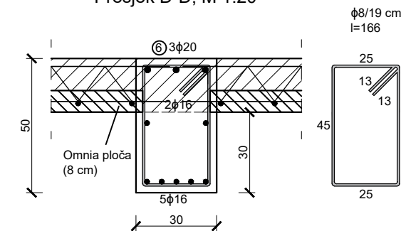
Presjek D-D, M 1:20
