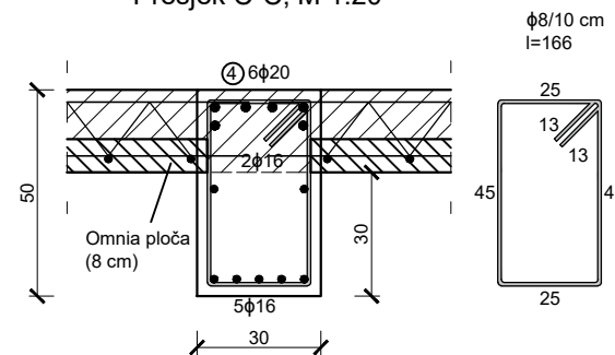
Presjek C-C, M 1:20
