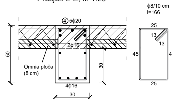
Presjek E-E, M 1:20
