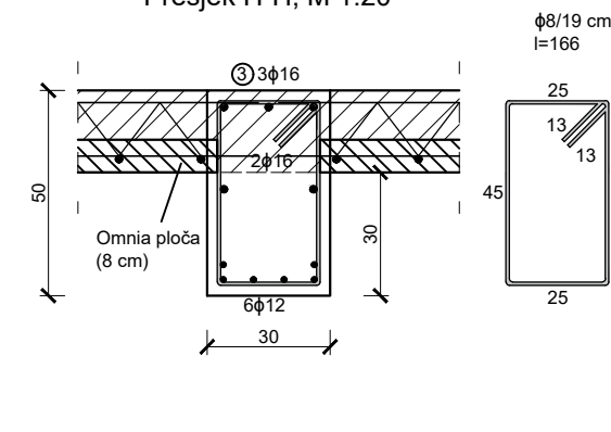
Presjek H-H, M 1:20
