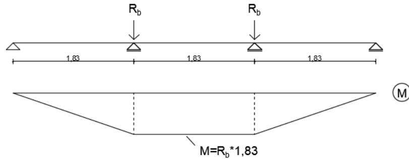
Slika 18: Statički sustav Omnia ploče u fazi 2
