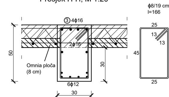
Presjek H-H, M 1:20
