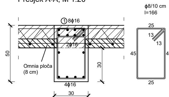
Presjek A-A, M 1:20
