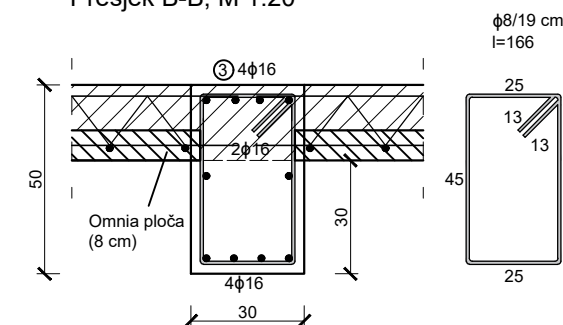
Presjek B-B, M 1:20
