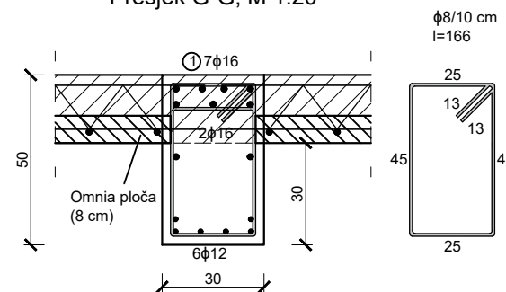
Presjek G-G, M 1:20
