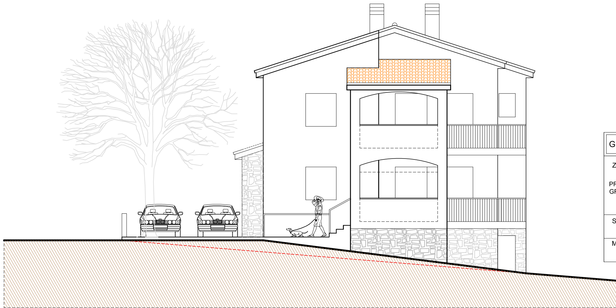
JUGOZAPADNO PROČELJE
