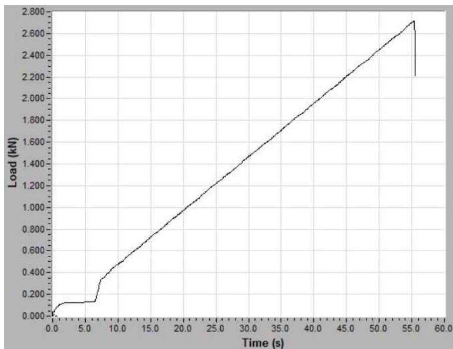
Slika 18. Karakteristični graf CM-PVC 30
