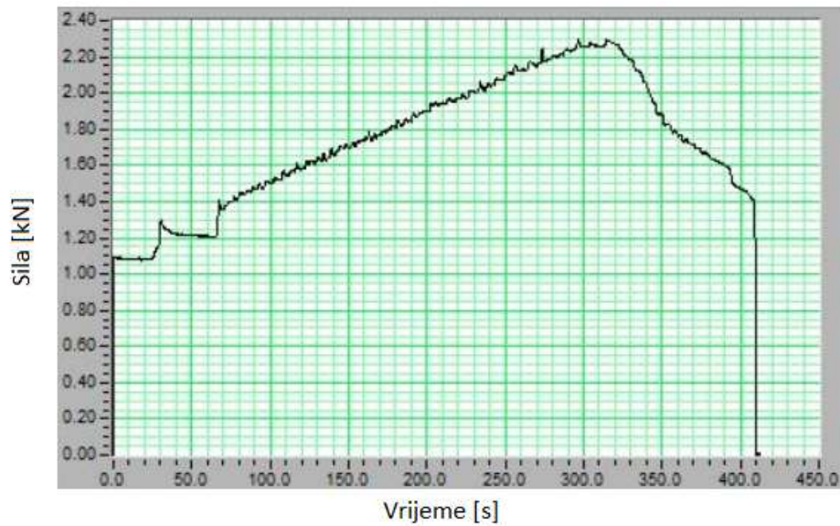
Slika 21. Karakteristični graf CM-PVC 30/pomak
