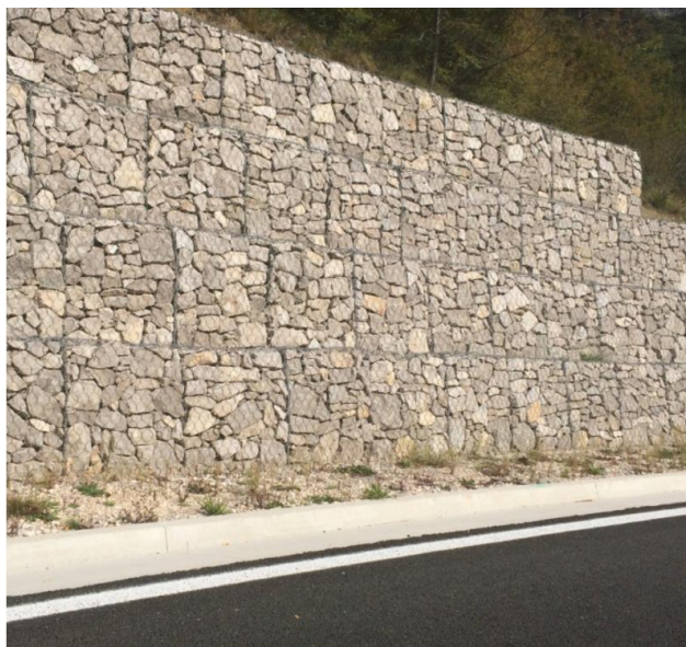
Slika 18 : Gabionski zid kraj autoceste A1 [18]
