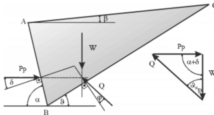
Slika 2 : Pasivni klin i poligon sila [15]
