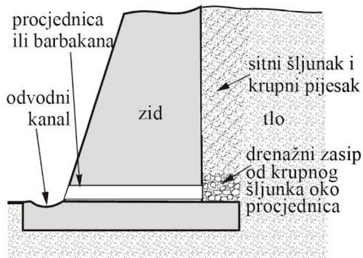
Slika 11 : Drenaža potpornog zida [16]
