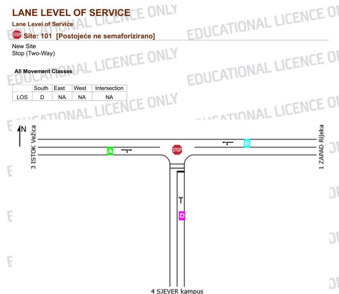
Slika 15. Razina uslužnosti za sadašnje stanje
