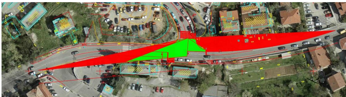
Slika 40. Preglednost SAD norme sporedni smjer skretanje u lijevo
