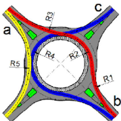
Slika 3. Putanja osobnog vozila za kontrolu proвозne brzine [3]
