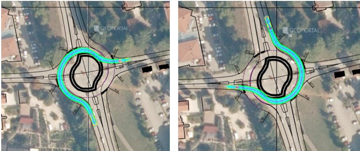
Slika 46. Provoznost - lijevi skretači sa sporednog smjera
