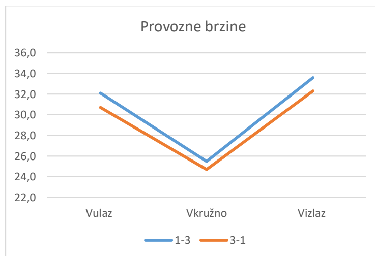
Slika 32. Varijantno rješenje 2 - provozne brzine
