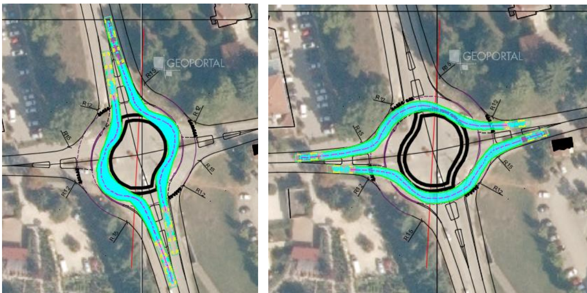
Slika 43. Provoznost - prolazak ravno
