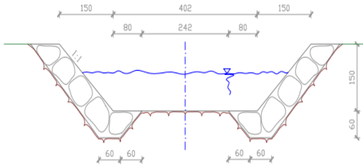
c) NORMALNI PROFIL KANALA OD 0+102,76 DO 0+122,40
