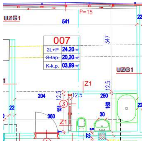
Slika 64: Soba 2L+P etaže sutereana -3 hotela Jadran (izvor: izvedbeni projekt (arhitektura) "Studia Remik" d.o.o.)
