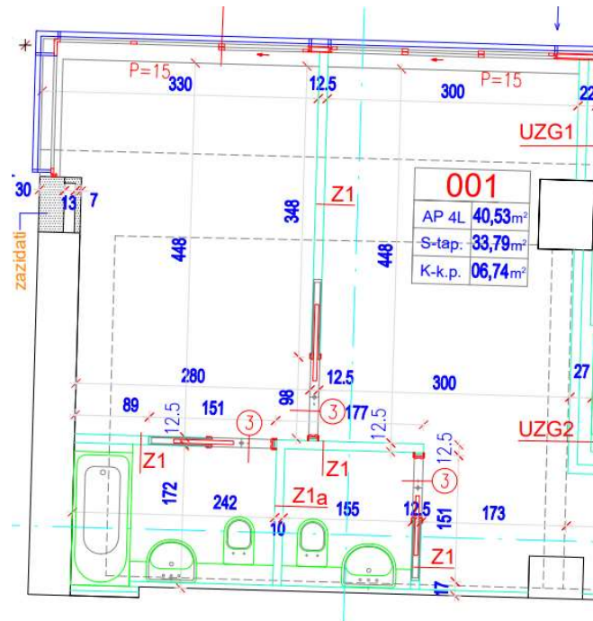
Slika 63: Apartman 4L etaže sutereana -3 hotela Jadran (izvor: izvedbeni projekt (arhitektura) "Studia Remik" d.o.o.)
