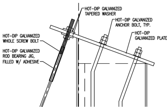
Slika 10: Detalj povezivanja šipke [7]
