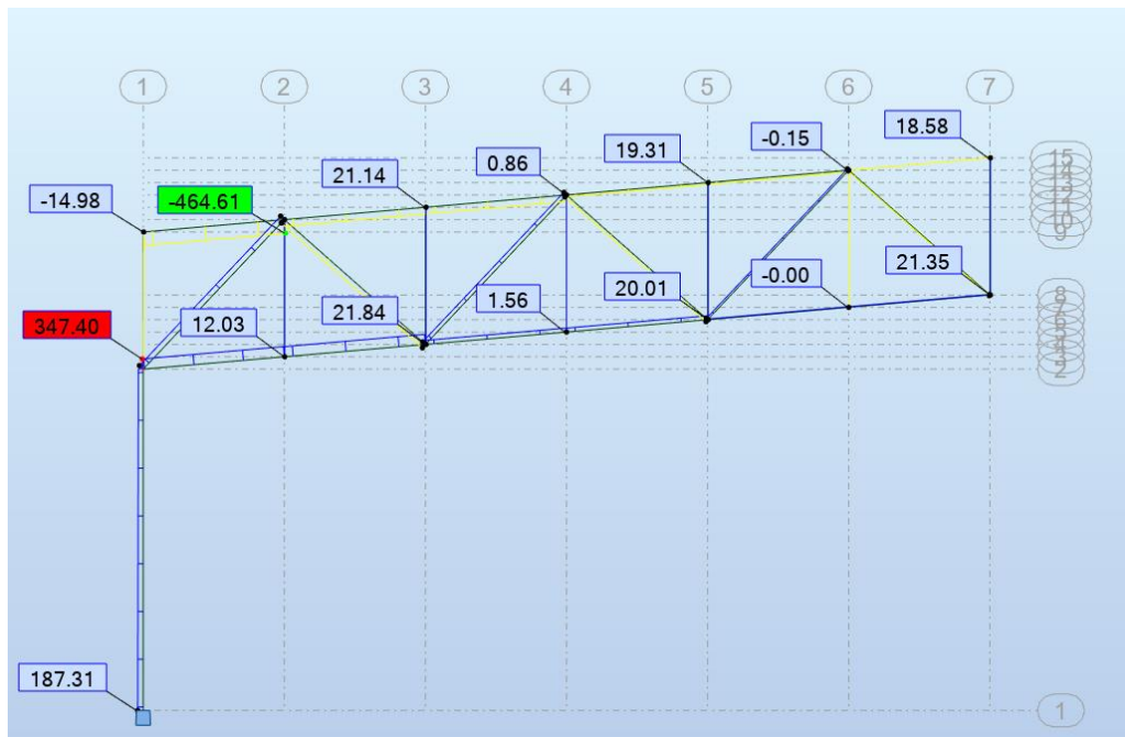
Slika 35: Dijagram uzdužnih sila u nosaču za pritiskajuće djelovanje
