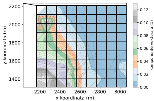
Slika 4.14 Grafički prikaz rasporeda očekivanih položaja gubitaka vode dobiven metodom korelacijskog koeficijenta za primjer D.
