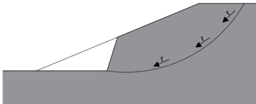
Slika 3. Rasterećenje dna kosine uzrokovano uklanjanjem potporne konstrukcije [5]
