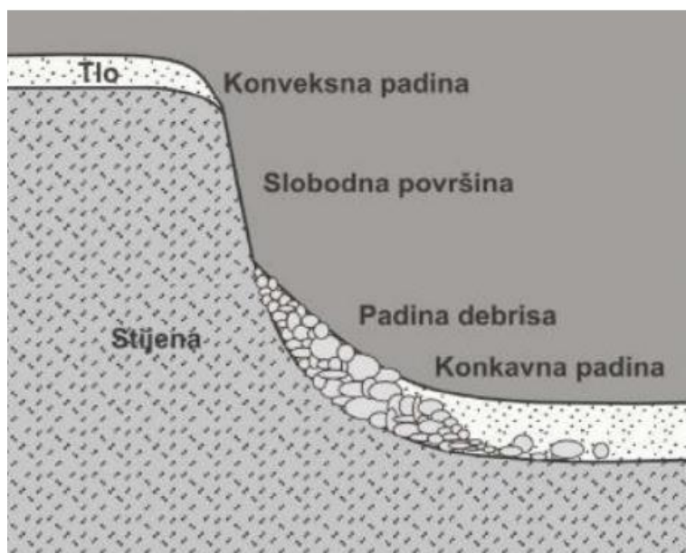
Slika 14. Elementi padine, konveksnost i konkavnost padine [16]
