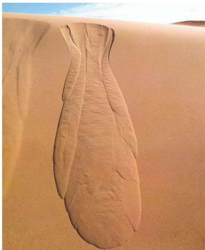
Slika 37. Tečenje suhog pijeska na padini pustinske dine, pustinja Namib [12]
