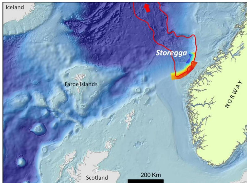
Slika 32. Lokacija i produžetak podvodnog klizišta Storegga, Norveška [28]
