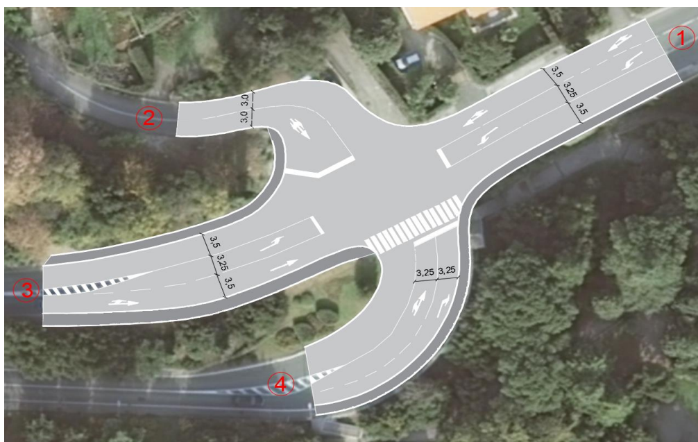
Slika 20: Prikaz raskrižja Vrutki s privozima
