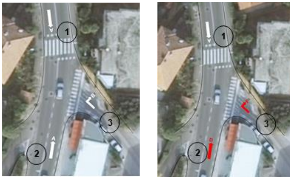
Slika 41: Razine uslužnosti za sve prilive i kretanja na raskrižju Tržnica prema vanezonskom (lijevo) i sezonskom (desno) prometnom opterećenju
