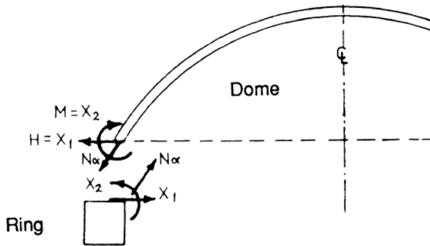
Slika 19: Interakcija između ljuške i vlačnog prstena [3]
