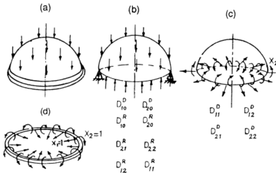
Slika 20: Metoda sila kod analize ljuške sa prstenom [3]
