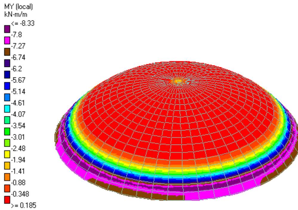
Slika 90: Model 3 - momenti savijanja u meridijalnom smjeru
