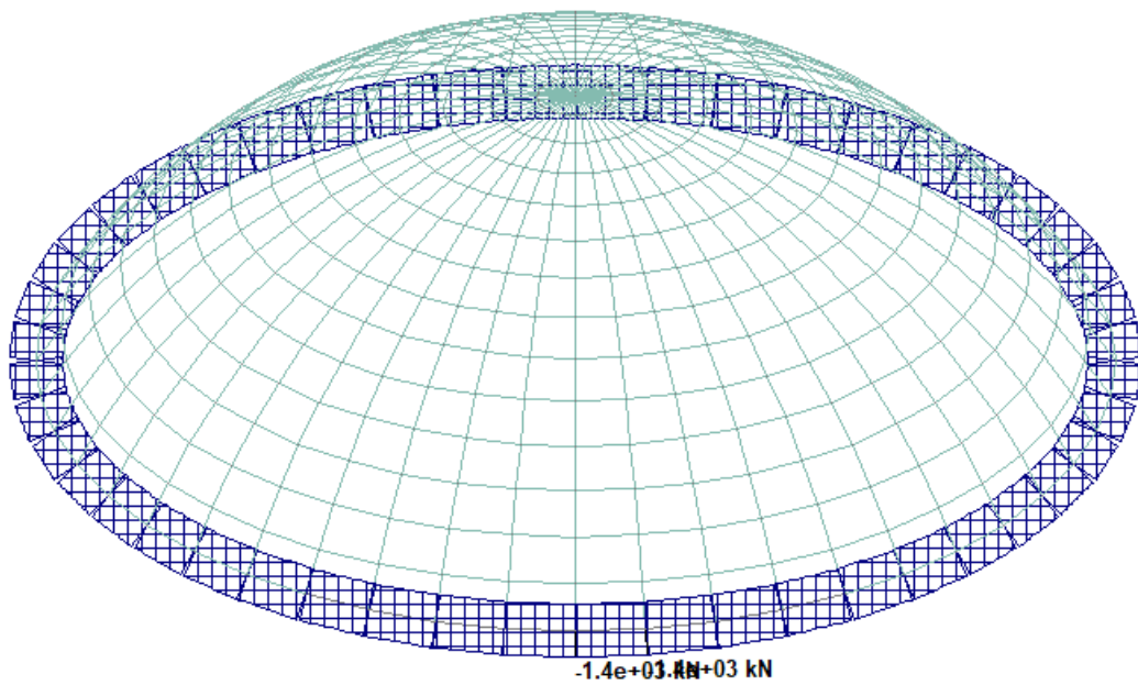
Slika 75: Model 1 - vlačna sila u prstenu (kombinacija opterećenja), F_x = 1398,17 kN
