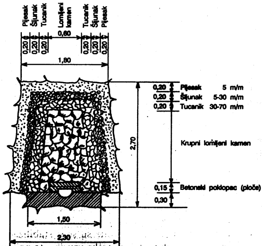
Slika 40. Drenažni potkop [8]
