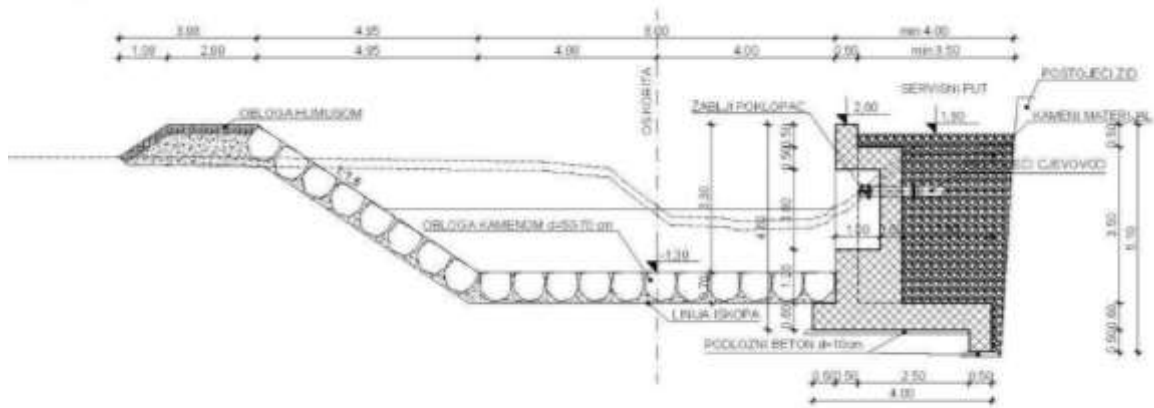
KARAKTERISTIČNI PRESJEK KROZ ISPUST M 1:100
