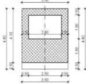
PRESJEK 1-1 M 1:100
