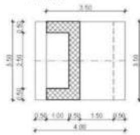
PRESJEK 2-2 M 1:100
