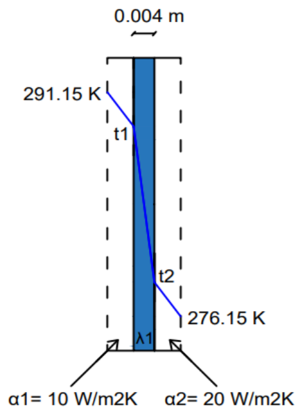
Slika 9: Shema za izračun prolaza topline kroz jednoslojnu staklenu stijenku pri noćnoj temperaturi
