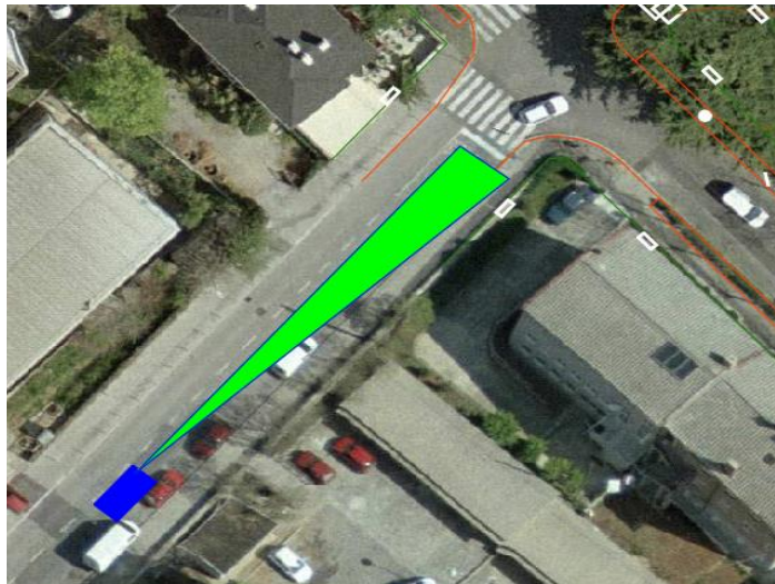
Slika 32: Zaustavna preglednost
