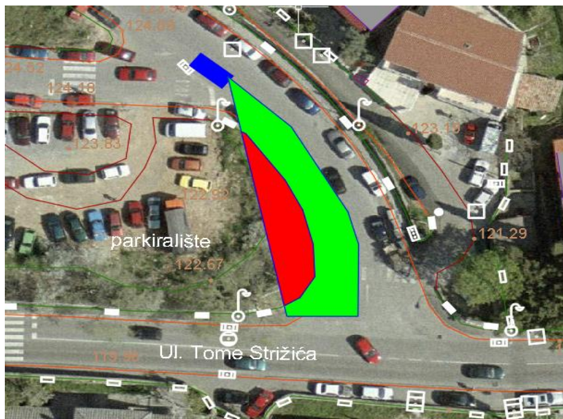
Slika 25: Zaustavna preglednost
