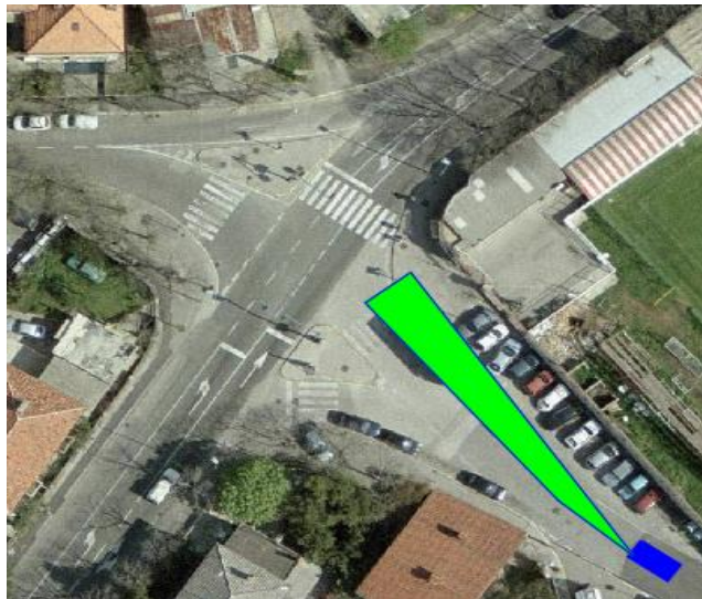
Slika 54. Zaustavna preglednost
