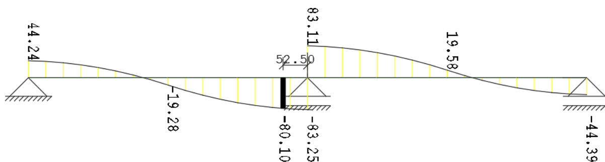
Slika 16. Dijagram poprečnih sila i reducirana poprečna sila uz ležaj B za središnju gredu poz.2
