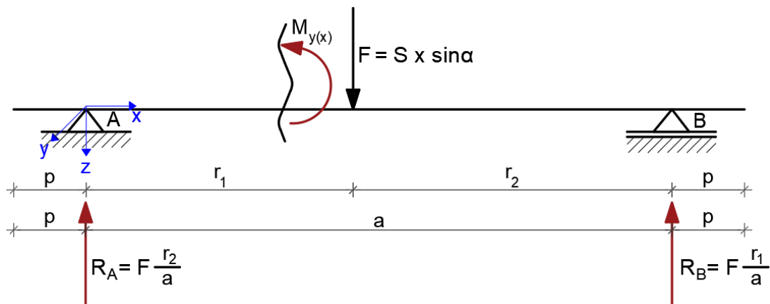
Slika 16: Greda opterećena samo silom F
