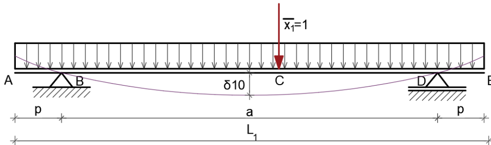
Slika 10: Osnovni sustav
