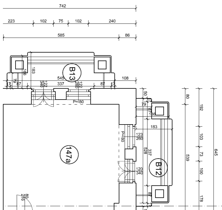
Slika 6 Dimenzije balkona
