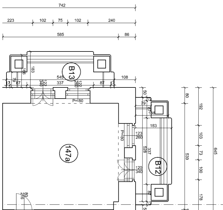
Slika 6 Dimenzije balkona
