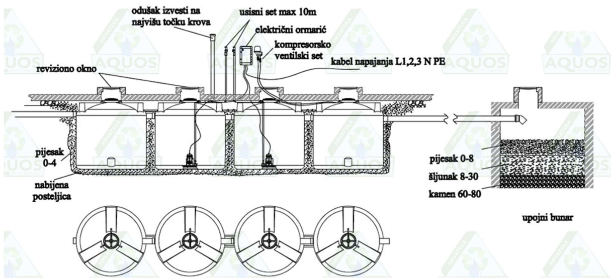
Slika 17: Primjer ugradnje biološkog pročištača
