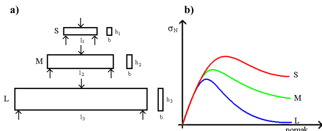
Slika 2. Tri geometrijski slične betonske grede opterećene na savijanje – (a) geometrija i (b) nominalna nosivost u funkciji pomaka mjerenoj na mjestu nanošenja opterećenja
