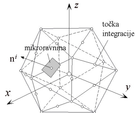
Slika 5. Koncept mikroravninskog modela: (a) komponente deformacija na mikroravnini i (b) tipična diskretizacija kugle jediničnog radijusa s dvadeset i jednom integracijskom točkom (simetrija)
