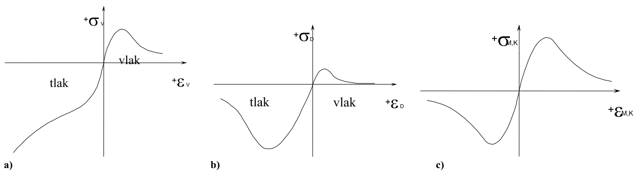
Slika 6. Veza između napreznja i deformacije (prikazana kvalitativno): (a) volumenska komponenta, (b) devijatorska komponenta i (c) posmične komponente, M i K
