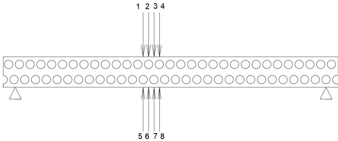
Slika 46: Lokacije tenzometra za model B2 LMD sa 15% ispune
