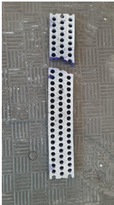
Slika 57: Puknuti uzorak B3 LMD sa 15% ispune
