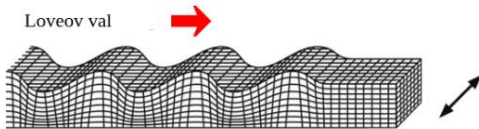
Slika 4 : Loveov val [5]
