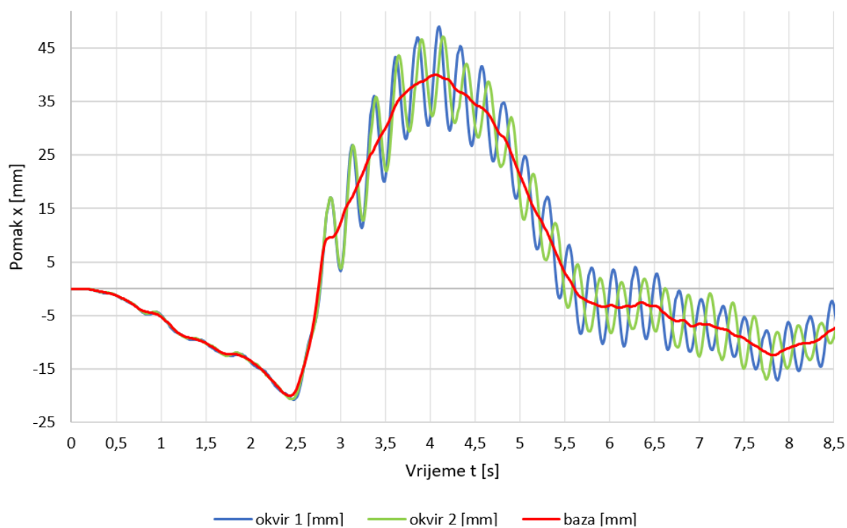
Slika 29 : Dijagram apsolutnih pomaka okvira izazvanih potresom „Cape Mendocino“
