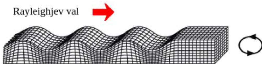
Rayleighjev val [5]
