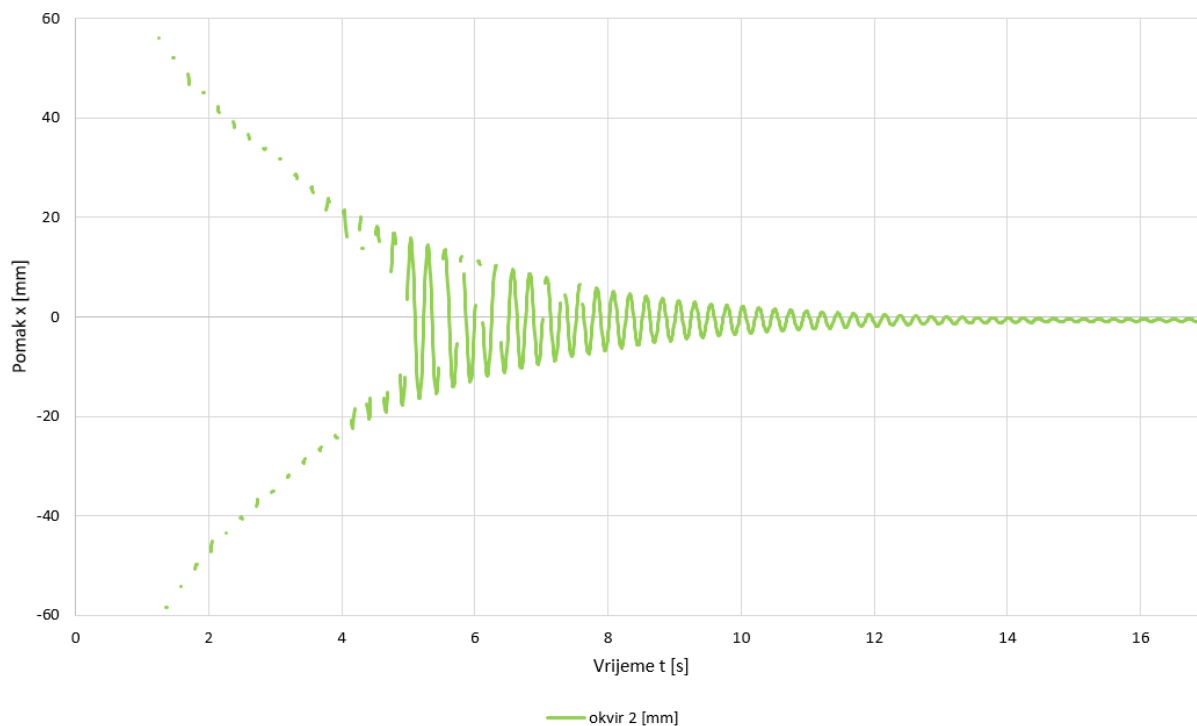
Slika 19 : Dijagram apsolutnih pomaka deformabilne ploče u vremenu
