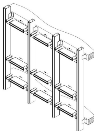
Slika 2: Tip montaže štapnog sustava vertikalno-horizontalno-vertikalno ( mullion-transom-mullion ); (Pripremio autor u programu Revit 2023 za potrebe ovoga rada)
