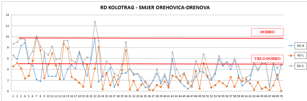
Slika 17. Dubine kolotruga na poddionicama za smjer Orehovica-Drenova
