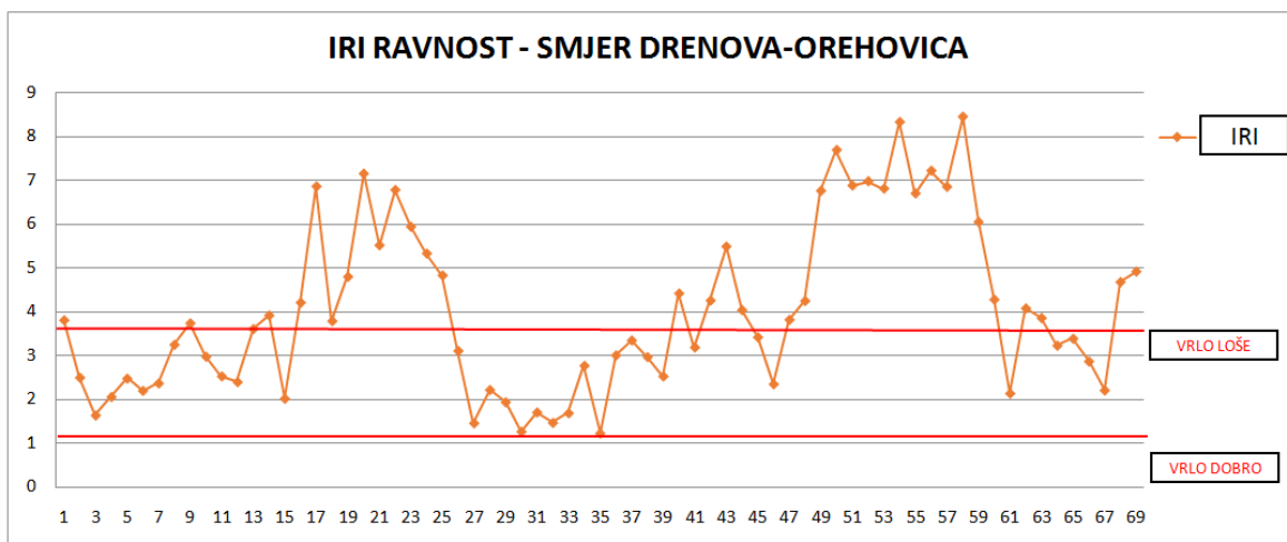
Slika 20. Ravnost IRI na poddionicama za smjer Drenova-Orehovica
