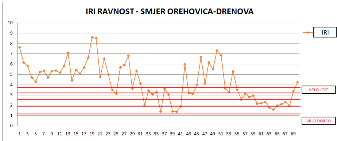
Slika 19. Ravnost IRI na poddionicama za smjer Orehovica-Drenova
