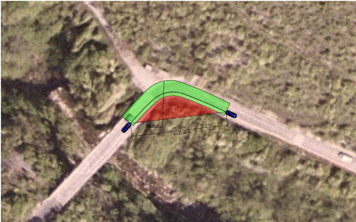
Slika 25. Preglednost horizontalne krivine R1 odabrane za analizu
