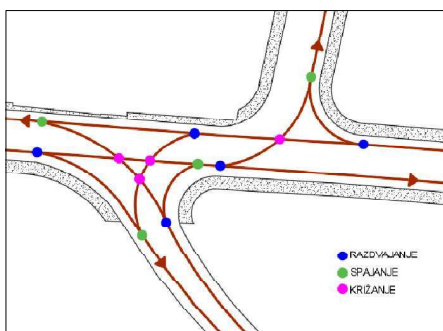
Slika 64. Konfliktnu točku na raskrižju 2 prema predloženim mjerama
