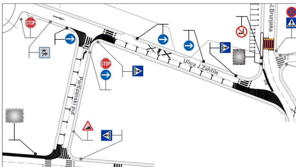
Slika 63. Prenamjena u jednosmjerne prometnice
