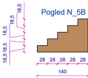
Pogled N_5B
