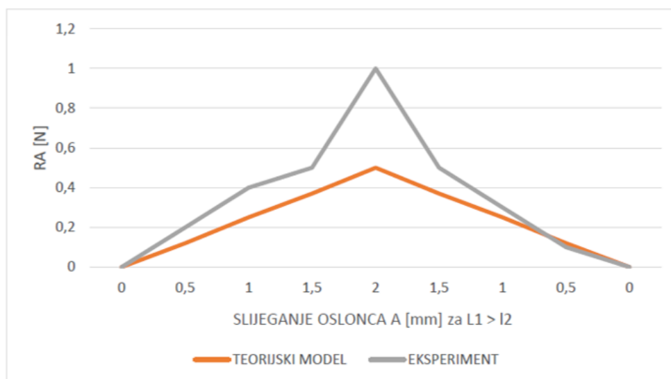
Slika 18: Grafička usporedba eksperimentalne i teorijske vrijednosti reakcije R_A za slučaj slijezanja oslonca A kada je L_1 > L_2
