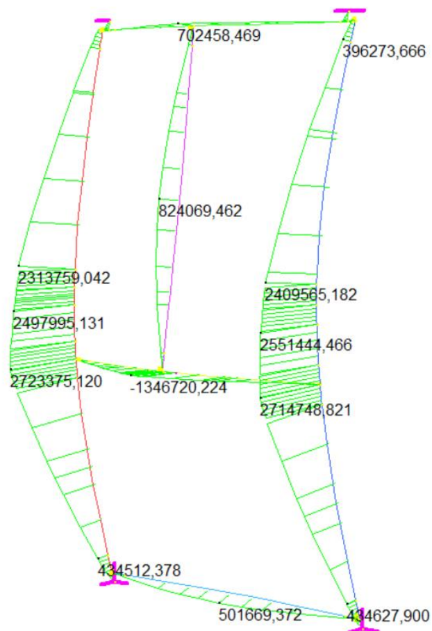
Slika 32. Vrijednosti momenata savijanja oko Y osi
