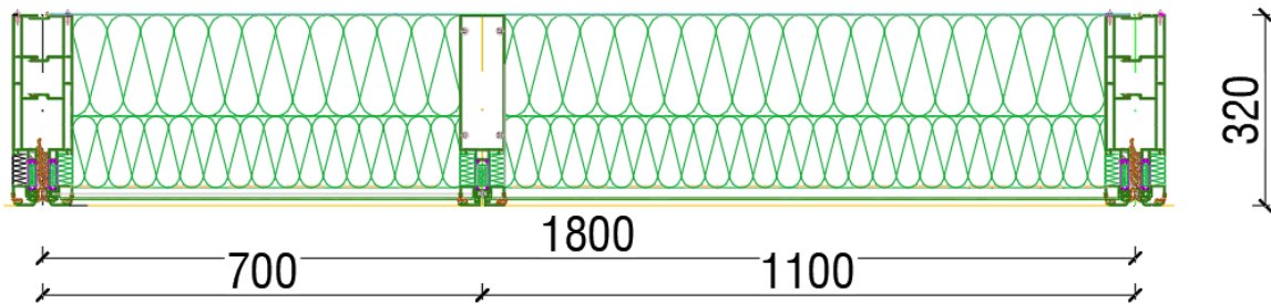
Slika 15. Horizontalni poprečni presjek fasadnog elementa
