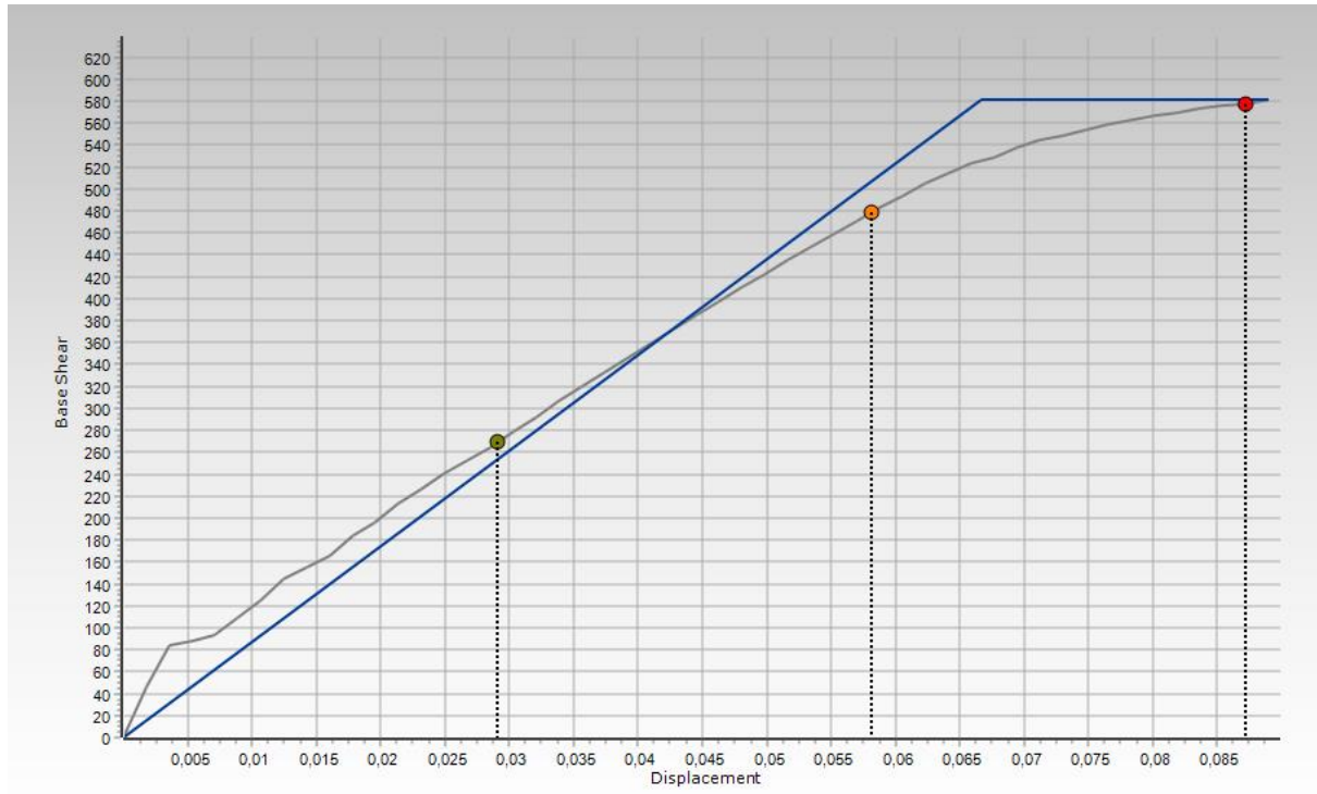
Slika 85: Krivulja sposobnosti po graničnim stanjima
