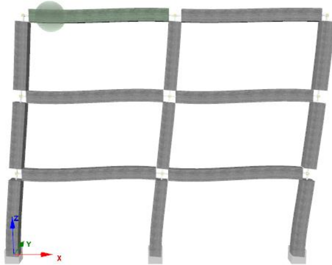
Slika 87: Plastični zglob na vanjskom osloncu grede POZ. 311
