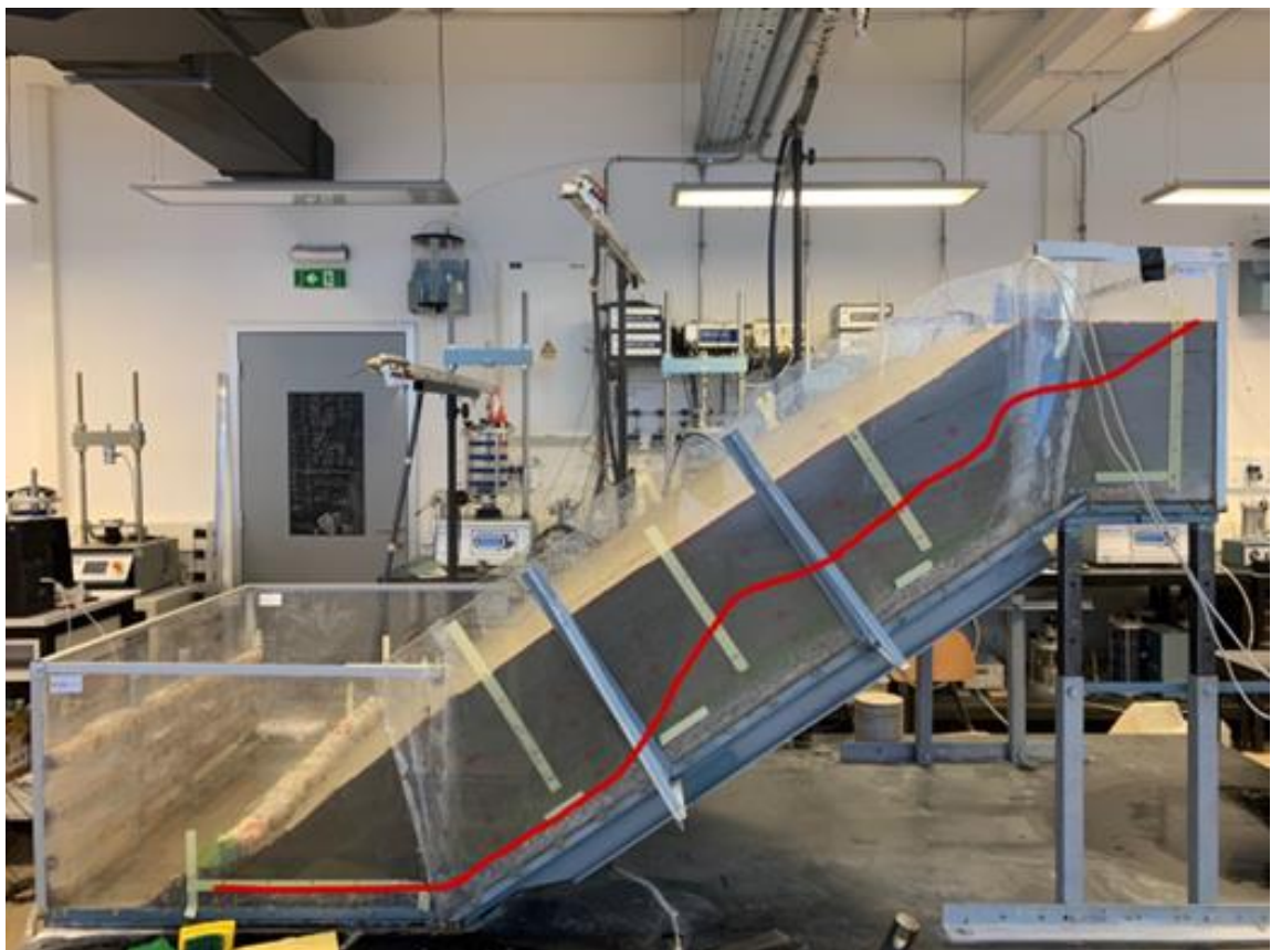
Slika 26. Prikaz prodiranja vode u materijal označen crvenom linijom.
