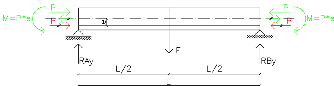
Slika 3. Spreng sila prednapinjanja
