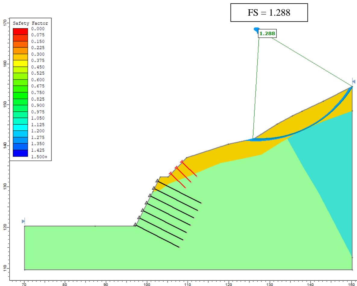
Slika 64. Model 3 – faktor sigurnosti i plohe sa FS < 1,30
