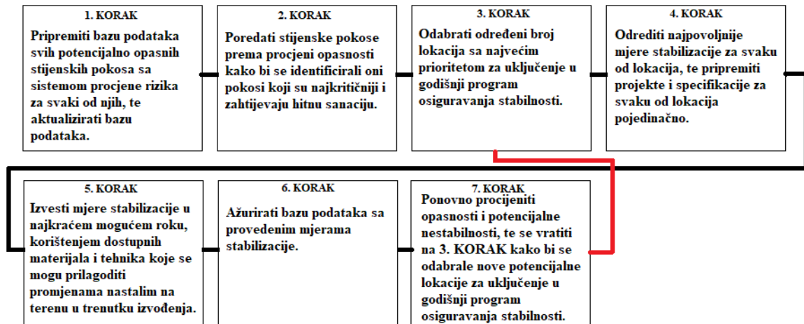
Slika 23. Stabilizacija stijenskog pokosa za transport (modificirano iz [2])
