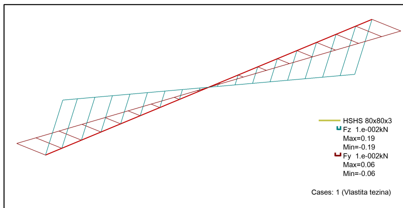
Slika 34: Dijagram poprečnih sila [kN]
