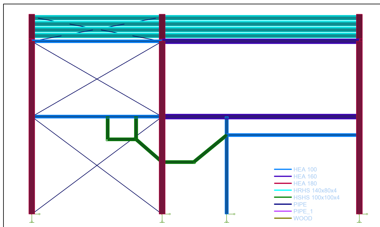
Slika 6: Stražnja fasada
