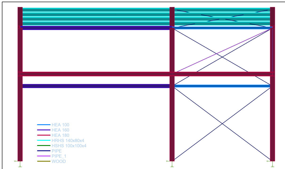
Slika 5: Ulazna fasada
