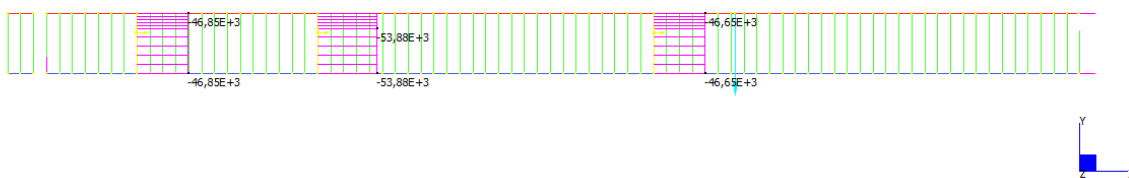
Slika 44. Poprečne sile na spajala grede A1 – model 1
